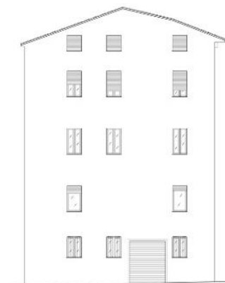
PROSPETTI SU PIAZZA D'AMICO - RAPP. 1:100
